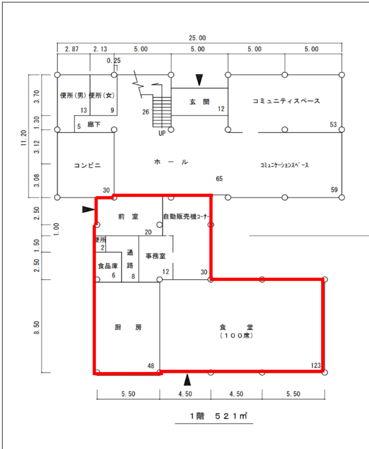
福利施設棟1階図面
