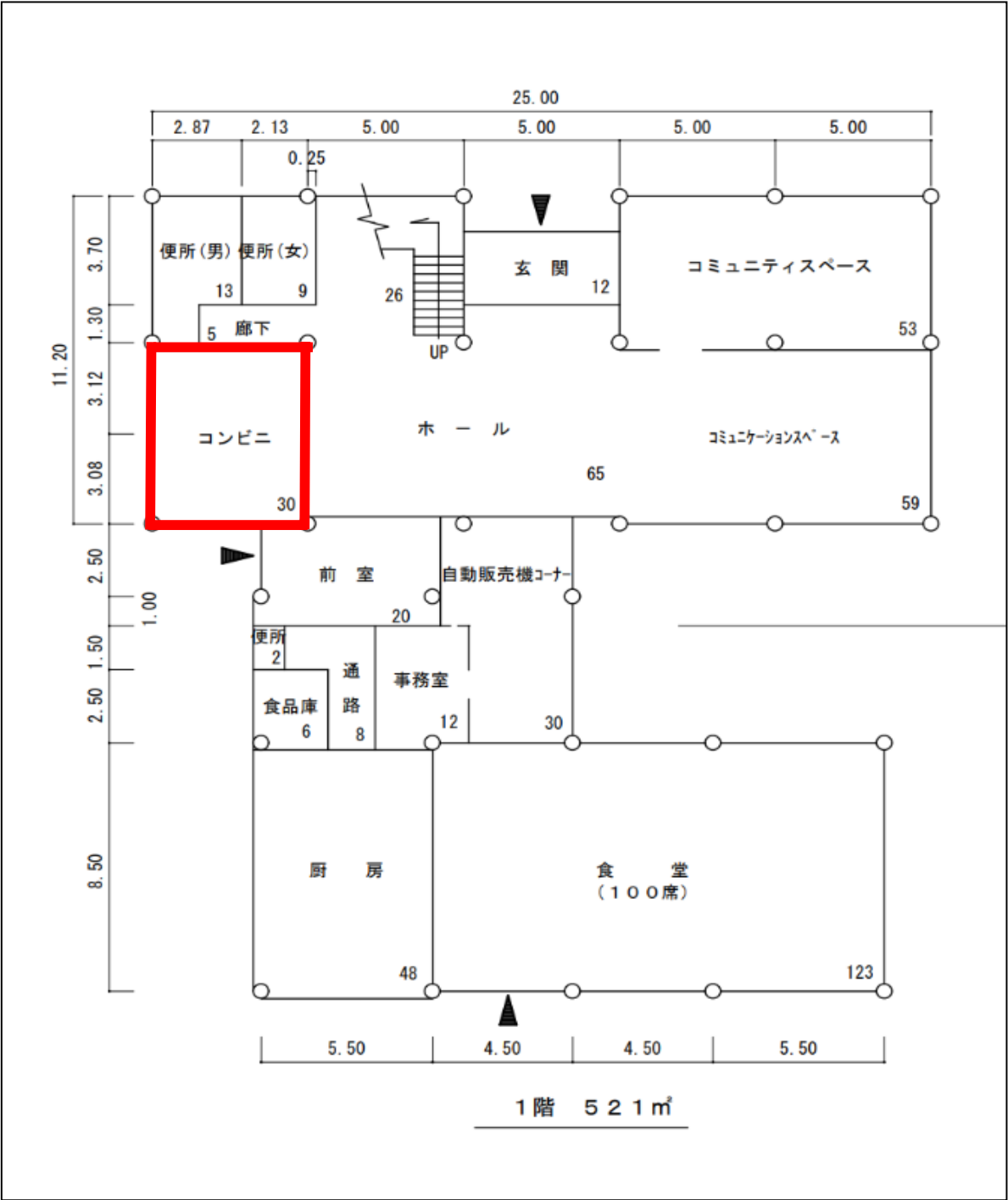
福利施設棟1階図面
