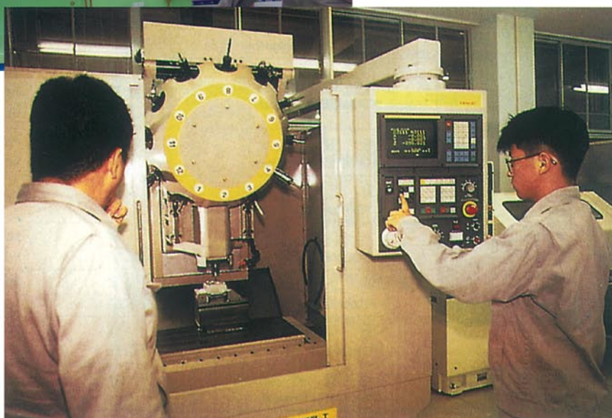
マシニングセンター装置による金型製作 Metal Mold Processing in the Machining Center
