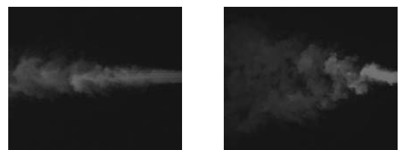
通常の噴流 往復振動流を付加した場合の噴流
