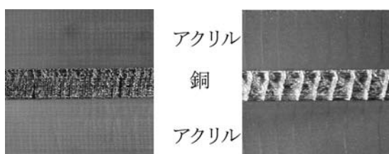
図1 加工条件の違いによる共削り加工面の違い
