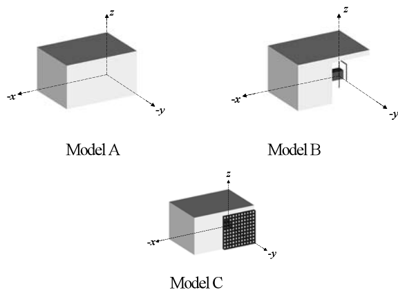
図1 比較モデル（1/8モデル）
