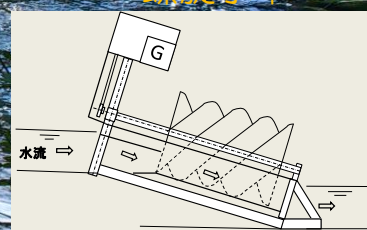
螺旋水車
