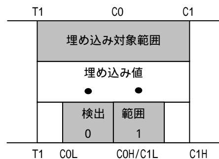
図 10 情報埋め込み・検出のしきい値
