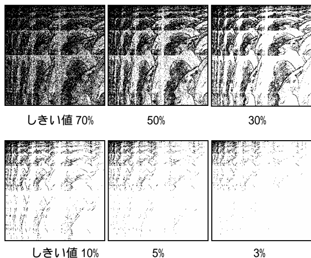
図 12 ウェーブレット変換 (Lena, Haar)
