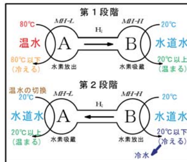
図2 冷却原理
