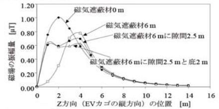
(b)磁気遮蔽材に底設置 磁界強度分布(x=3,000,y=0)解析結果 Bx成分(水平方向)
