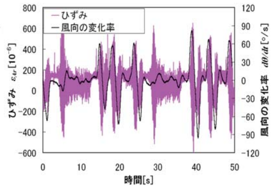
風向の変化率とひずみ波形
