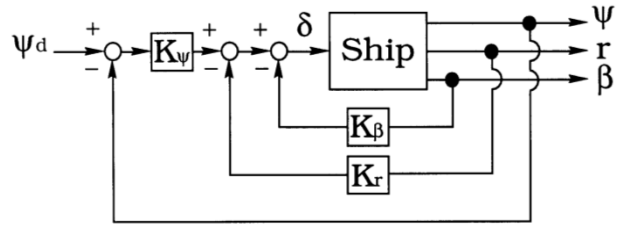
図2 制御系
