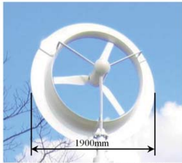
風レンズ風車 定格出力1kW 九州大学応用力学研究所内
