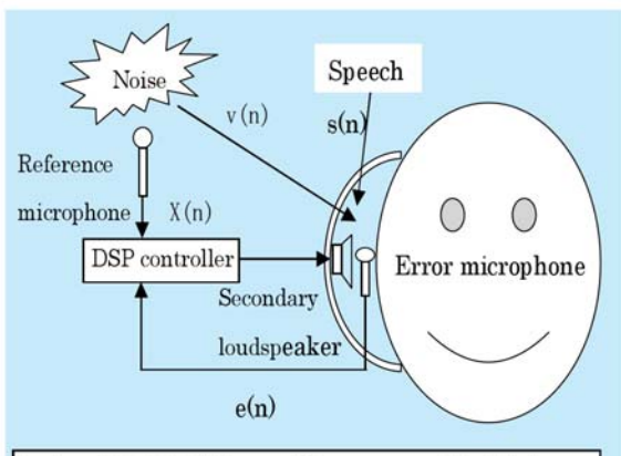
図1 騒音低減ヘッドフォンの構成図
