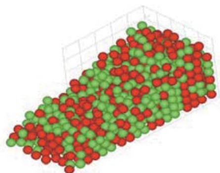
図4 個別要素法によるシミュレーション結果(3次元表示)
