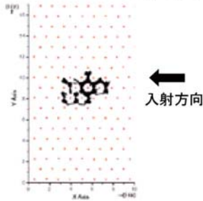
図1 X方向入射・入射角度 10^\circ ]の表面拡散の様子
