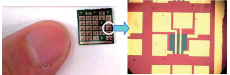
学生実験で作製したnMOS NAND回路
