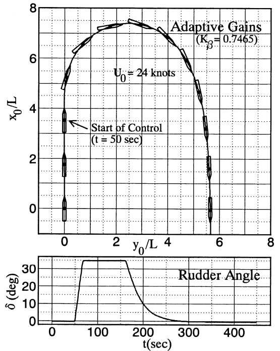
図3 適応ゲインを用いた時の旋回航跡
