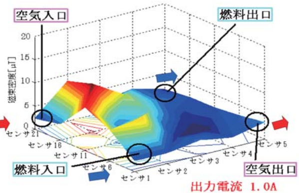
図4 開発システムによる発電磁場計測結果
