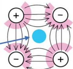
電気四重極による電界の様子
