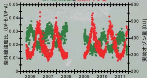
紫外線強度比と実効オゾン量
