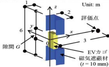
(a)磁気遮蔽材に隙間設置 解析モデル(1/2モデル)
