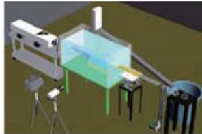
図3. 実験装置
