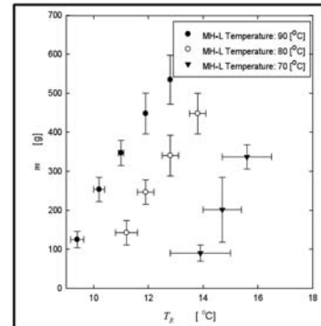
図3 冷却性能
