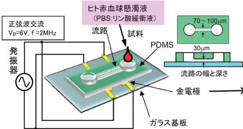
平面電気四重極
