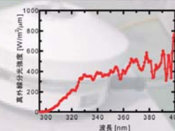
紫外線のスペクトル観測
