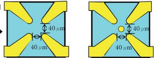
平面電気四重極
