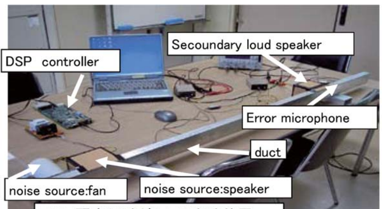
図2 騒音低減ダクトの実験装置
